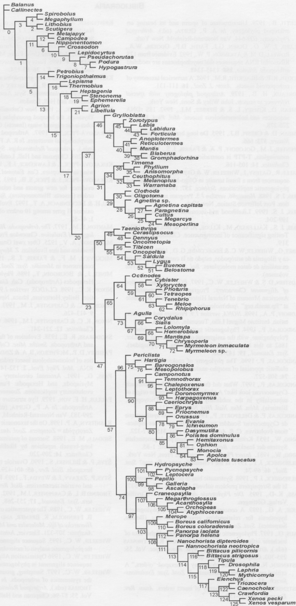
Fig. 4. - Relaciones de los hexápodos basadas en el análisis simultáneo de caracteres morfológicos y moleculares, como se describe en el texto y en Wheeler et al. (1999). Los números de los nodos bajo las ramas hacen referencia a los valores de soporte de Bremer en Wheeler et al. (1999: tabla 4).
