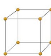
cubic
