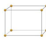
orthorhombic
